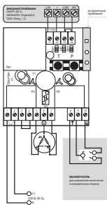
Рис. 3. Схема подключения двигателя рольставни и внешнего радиуправления к DoorHan CV01
